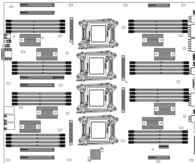
图 1-6 主板示意图
